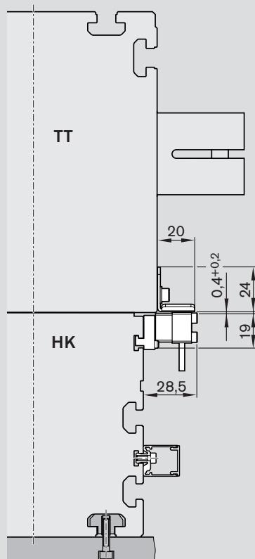
Interruptores inductivos con elementos de montaje / canal portables
